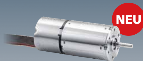
FAULHABER BX4 IMC BÜRSTENLOSE DC-SERVOMOTOREN MIT INTEGRIERTEM MOTION CONTROLLER
